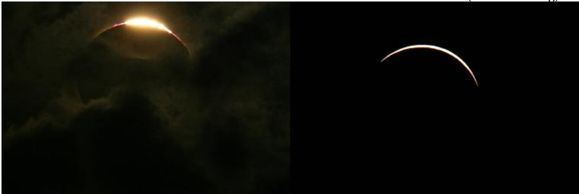
08:36:39 UT (Diamond Ring)
